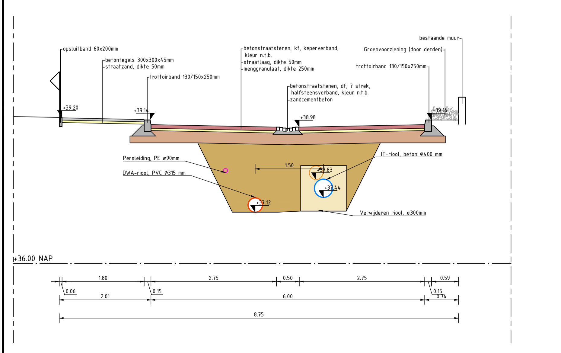
Doorsnede G-G: Bremlaan Schaal 1:50
