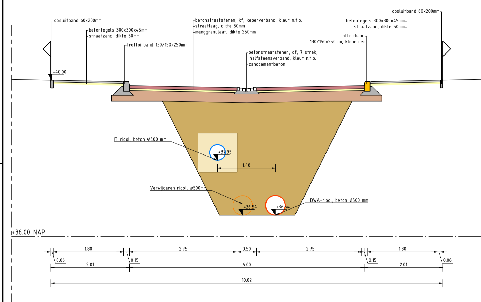
Doorsnede D-D: Clematislaan Schaal 1:50
