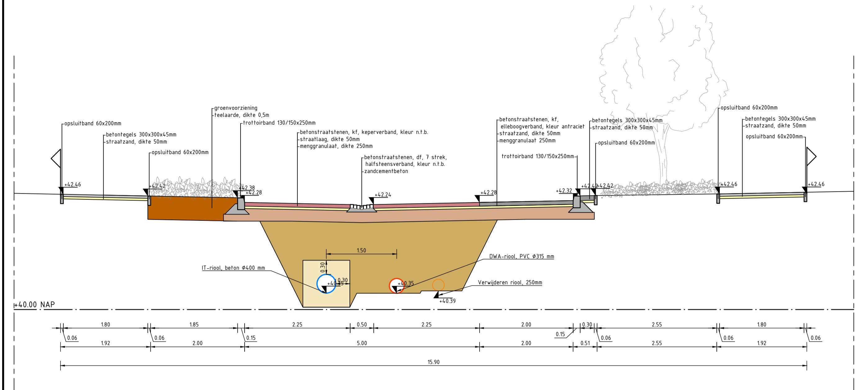
Doorsnede A-A: Beukenlaan Schaal 1:50
