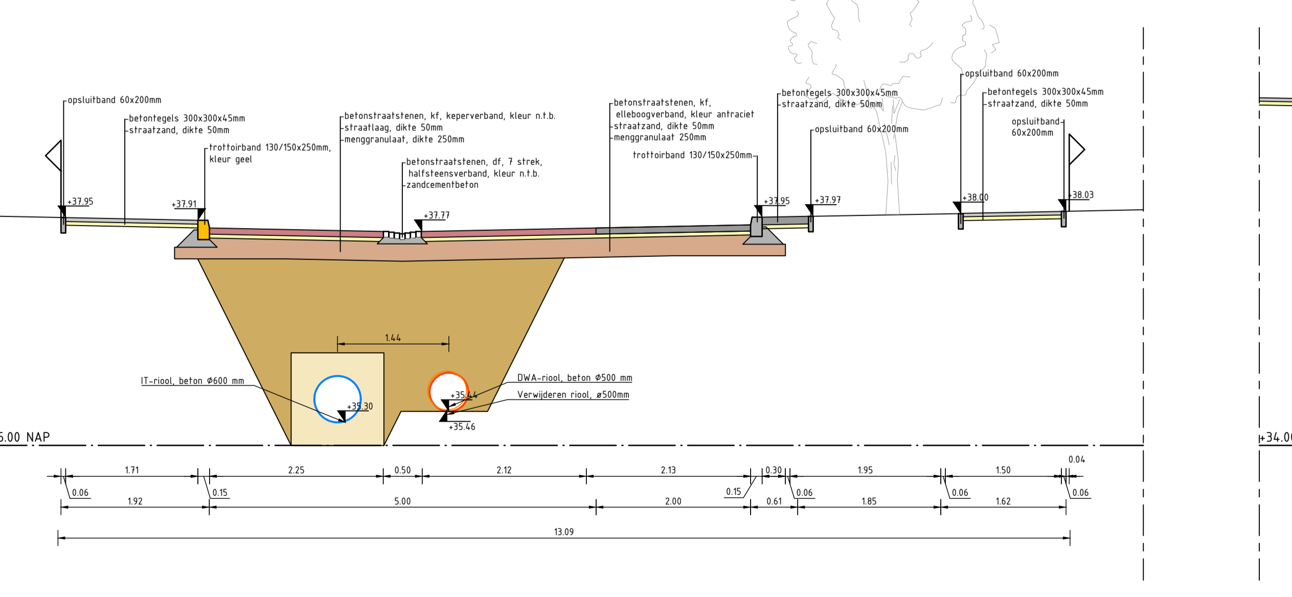
Doorsnede H-H: Beukenlaan Schaal 1:50
