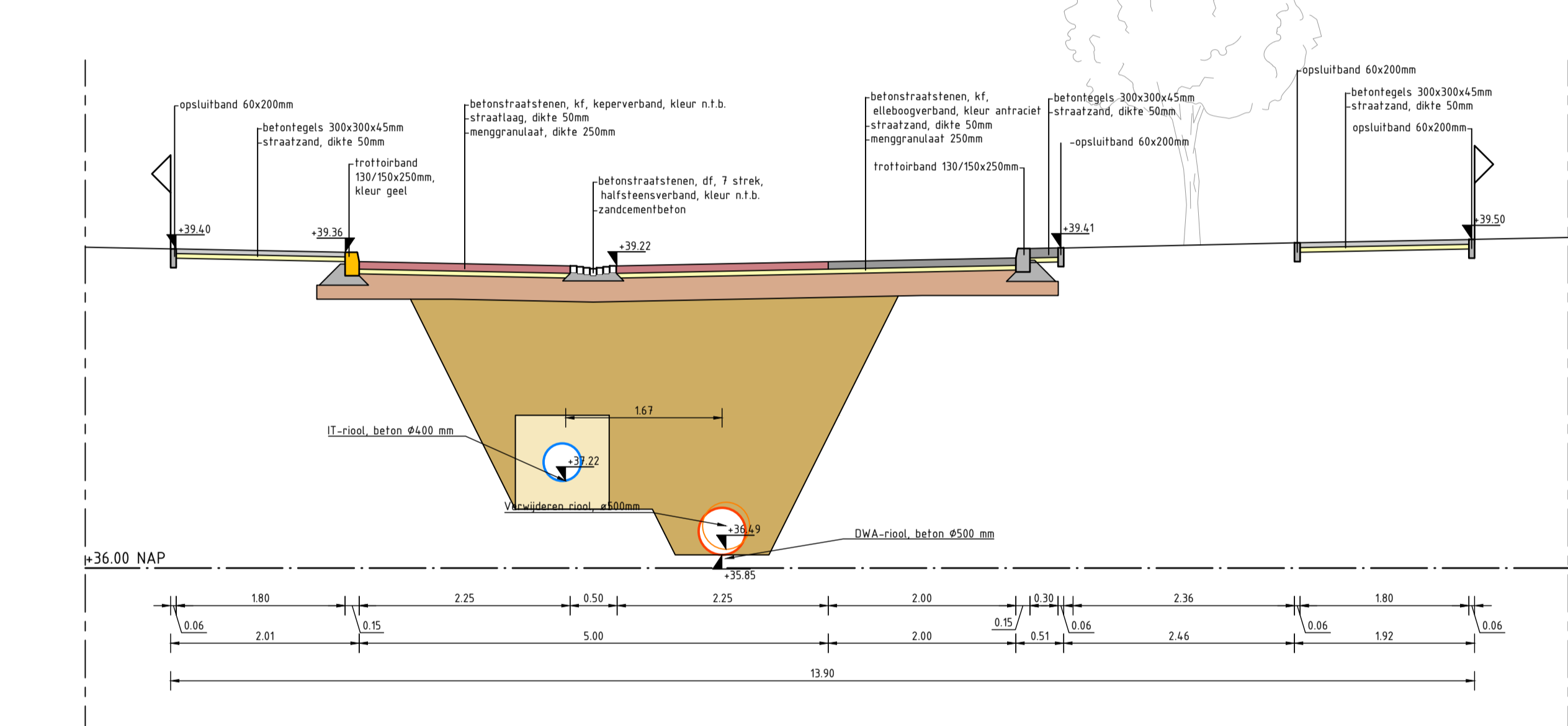
Doorsnede E-E: Ericalaan Schaal 1:50
