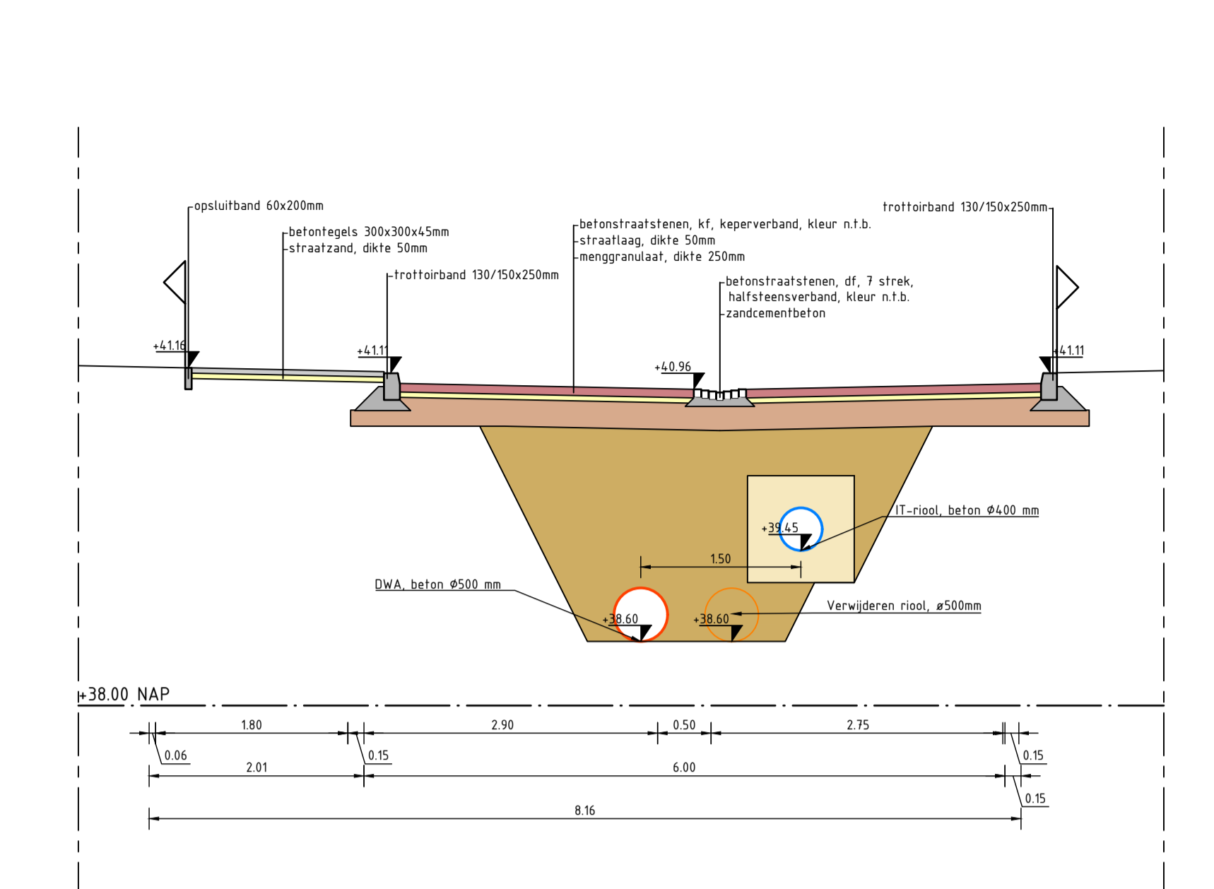
Doorsnede C-C: Bremlaan Schaal 1:50
