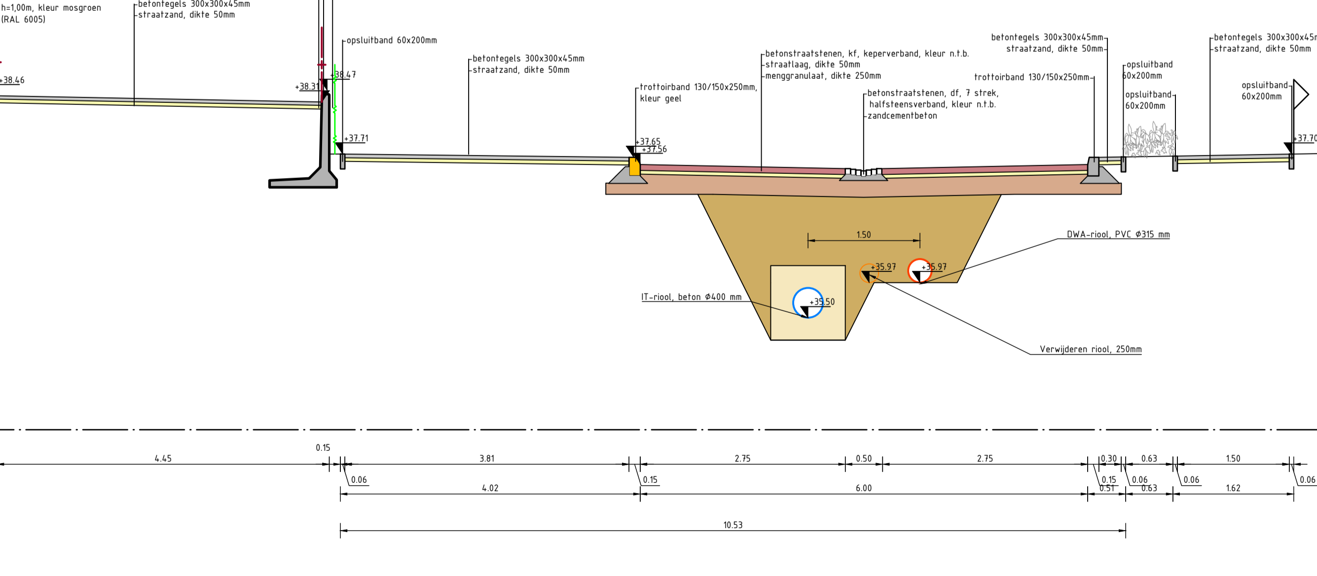
Doorsnede I-I: Ericalaan Schaal 1:50
