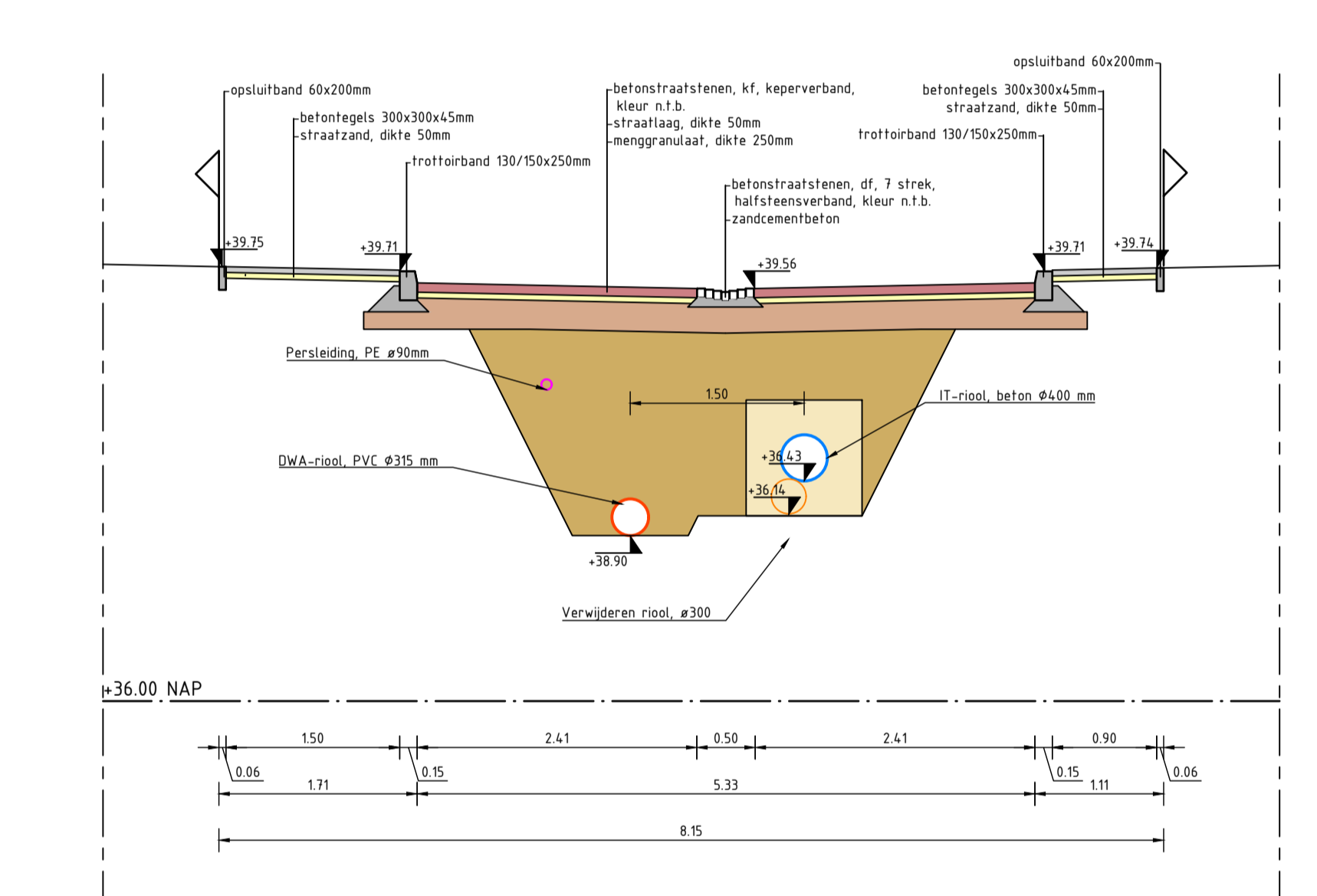
Doorsnede F-F: Bremlaan Schaal 1:50
