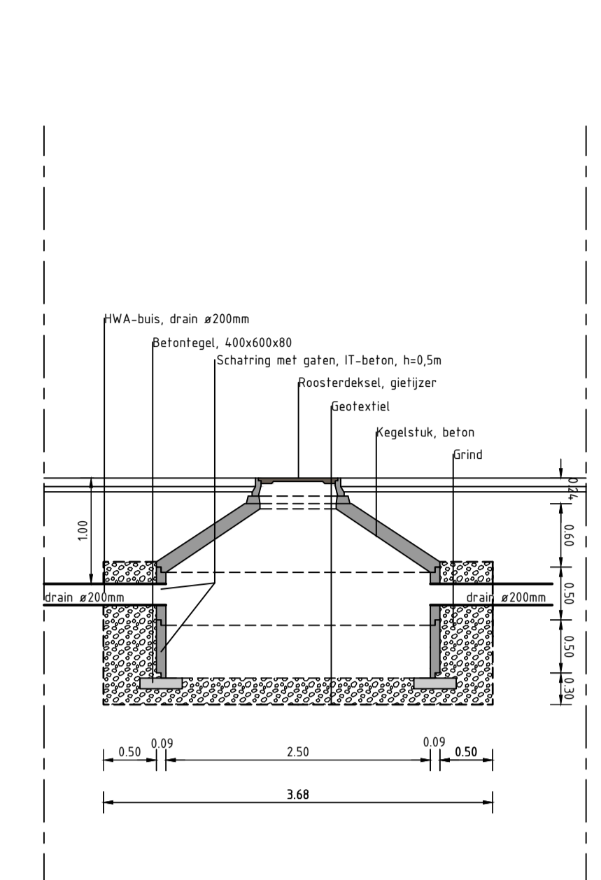
Principeddoorsnede; infiltratieput Schaal 1:50
