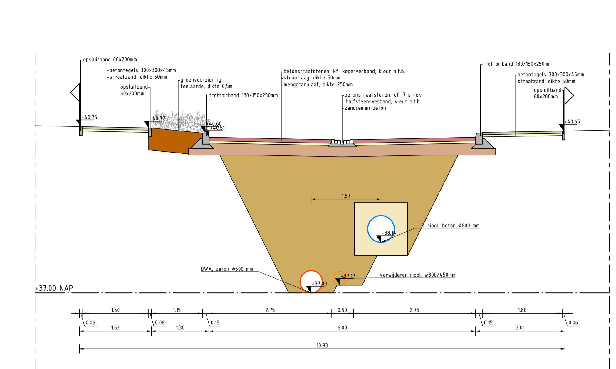
Doorsnede B-B: Ericalaan Schaal 1:50
